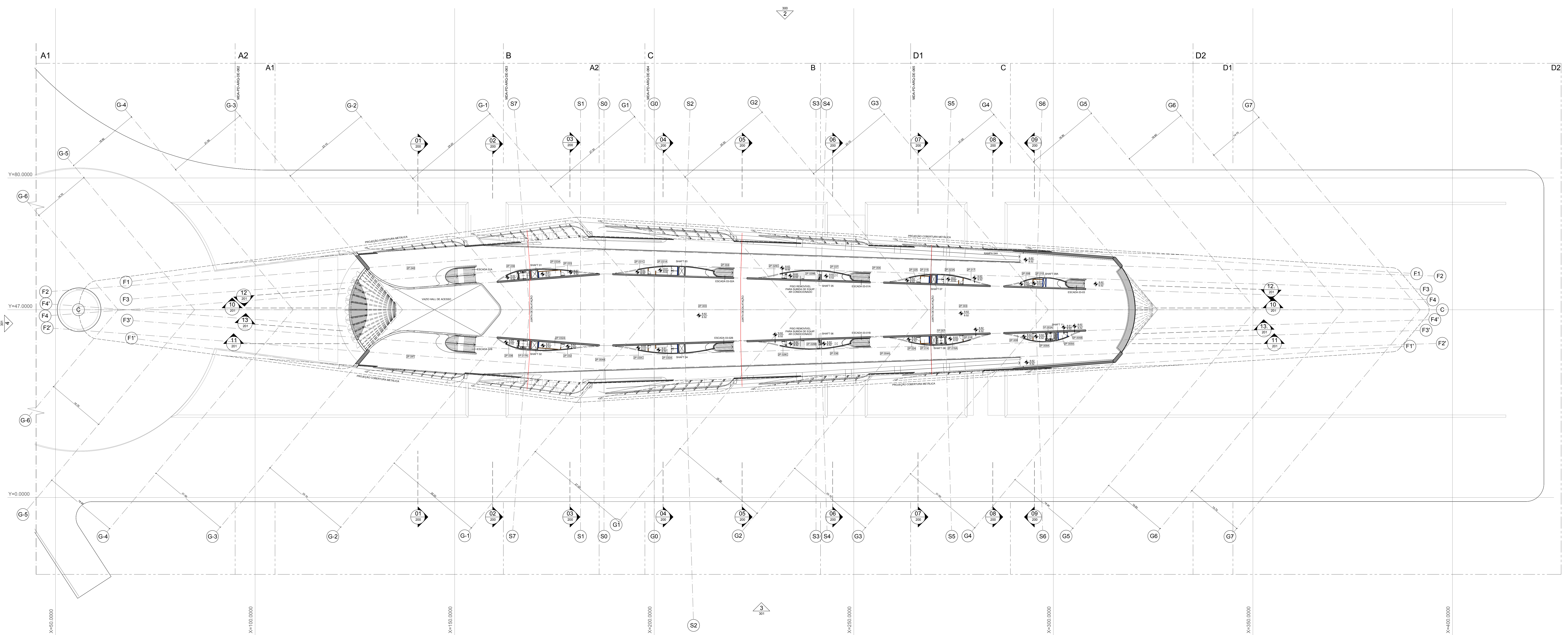
2º PAVIMENTO - PLANTA GERAL (NÍVEL +9.82) ESCALA: 1:300
